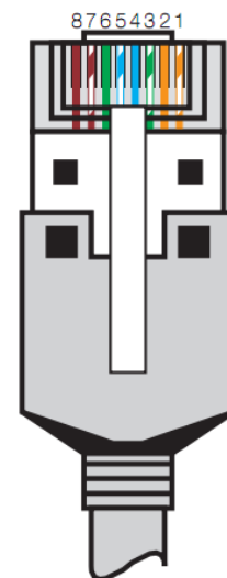
Abbildung 5: Steckverbinder RJ45
